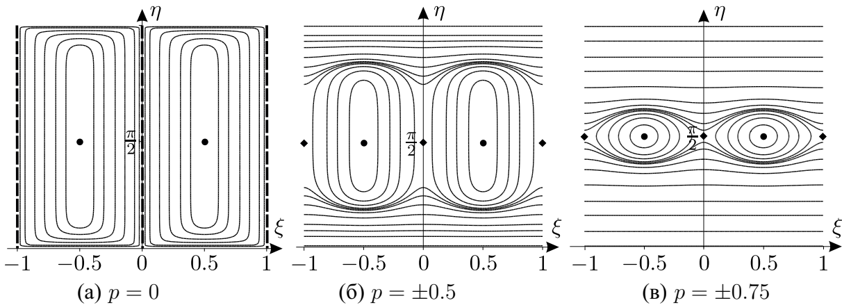
Рис. 2. Фазовые портреты при R = 1
