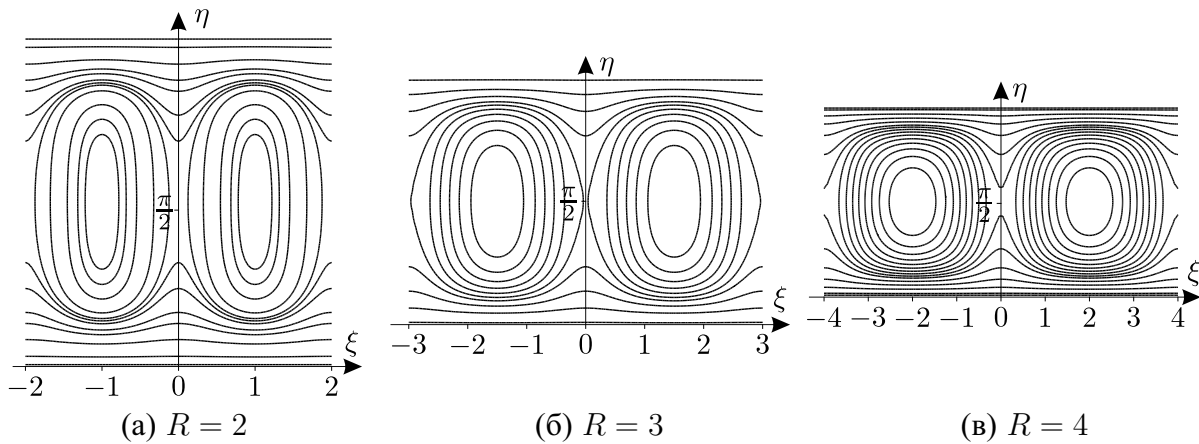
Рис. 4. Фазовые портреты при p = 0.5 и разных значениях R
