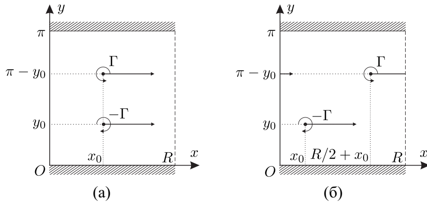
Рис. 3. Движения вихрей, соответствующие неподвижным точкам
