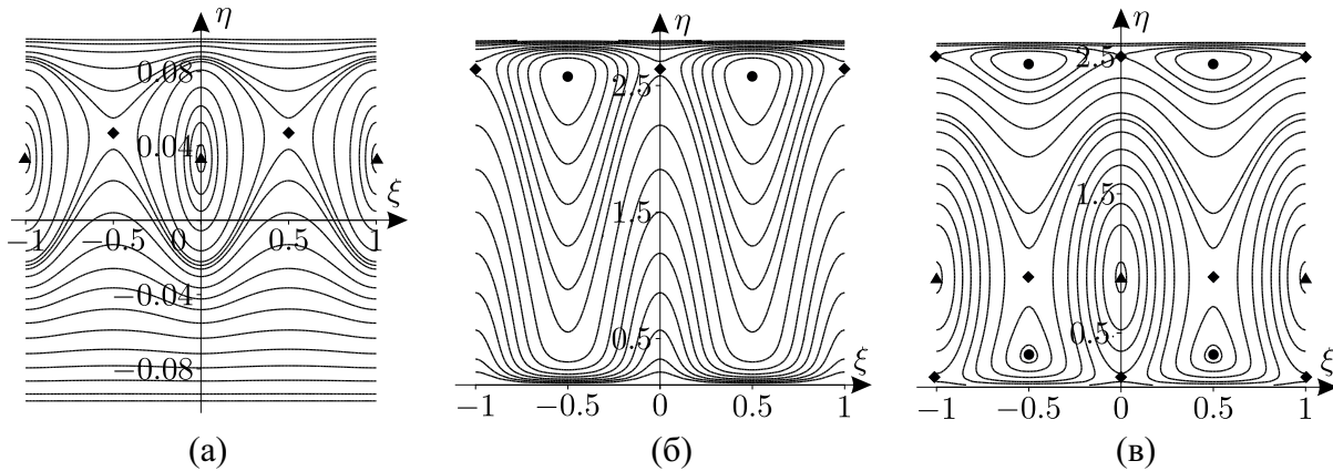
Рис. 7. Фазовый портрет при R = 1 и разных значениях параметров p, \gamma_1, \gamma_2
