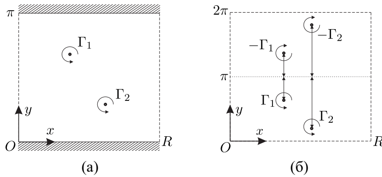
Рис. 1. Схематичное изображение вихрей: (а) на цилиндре, (б) на торе
