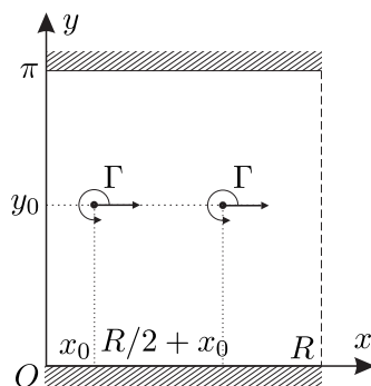
Рис. 6. Движение вихрей, соответствующее неподвижной точке
